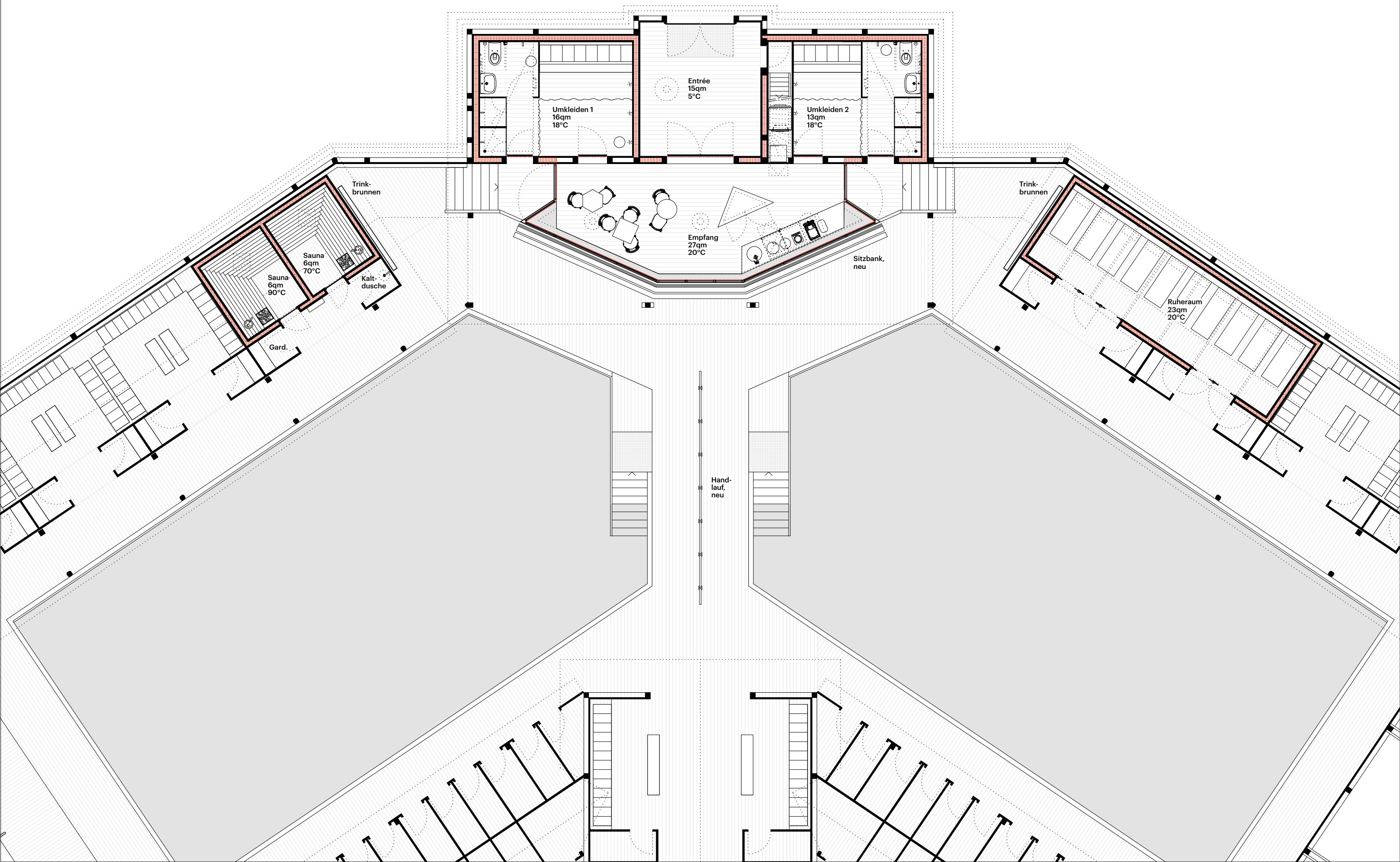
Grundriss Erdgeschoss 1:100
